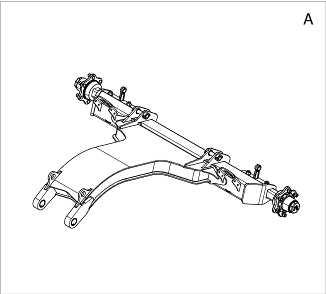
Hydraulic axle Hydraulická naprava
