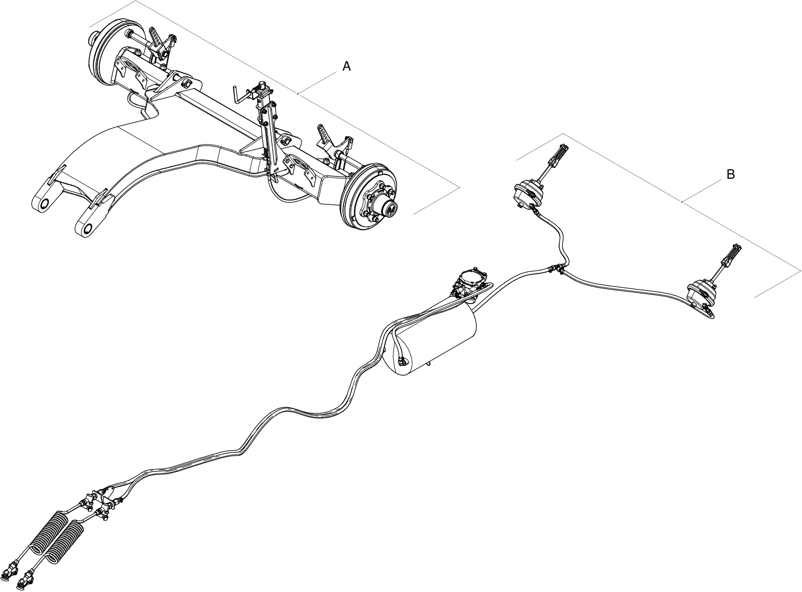
Achse mit Bremsen B
