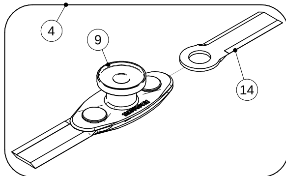
DOUBLE CHOPPER FRONT TRINCIA DOPPIO ANTERIORE DOPPEL HÄCKSLER VORDERSEITE
