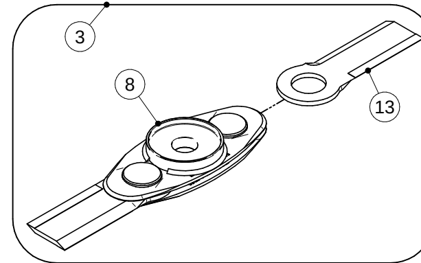
DOUBLE CHOPPER 22" REAR TRINCIA DOPPIO 22" POSTERIORE DOPPEL HÄCKSLER 22" RÜCKSEITE
