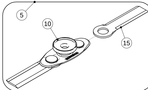
SINGLE CHOPPER TRINCIA SINGOLO EINZEL HÄCKSLER
