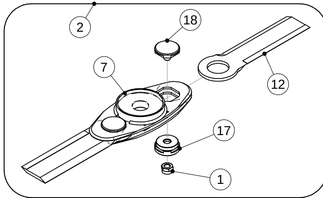
DOUBLE CHOPPER REAR TRINCIA DOPPIO POSTERIORE DOPPEL HÄCKSLER RÜCKSEITE
