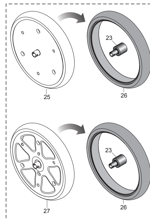
2" «V» SHAPED RUBBER PRESS WHEEL
