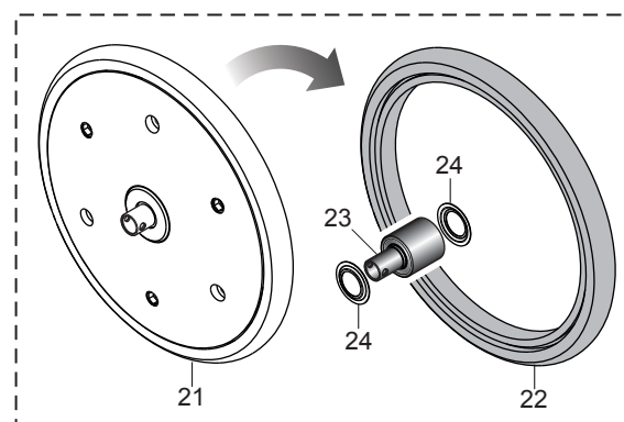
1" «V» SHAPED RUBBER PRESS WHEEL
