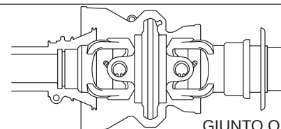
GIUNTO OMOCINETICO CONSTANT VELOCITY JOINT
